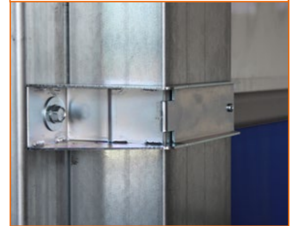
Verstärkungswinkel für höheren Windlastklasse
